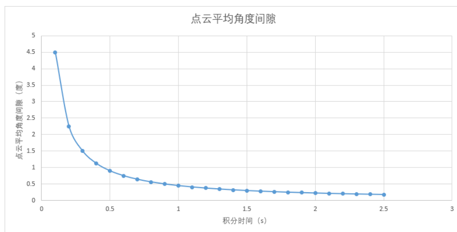
LDS-M300-E-3 不同积分时间点云平均角度间隙
