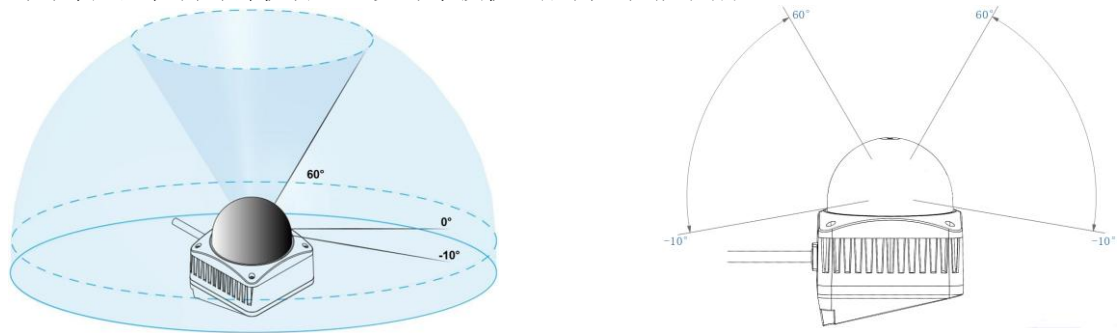
LDS-M300-E-3 有效 FOV 范围
