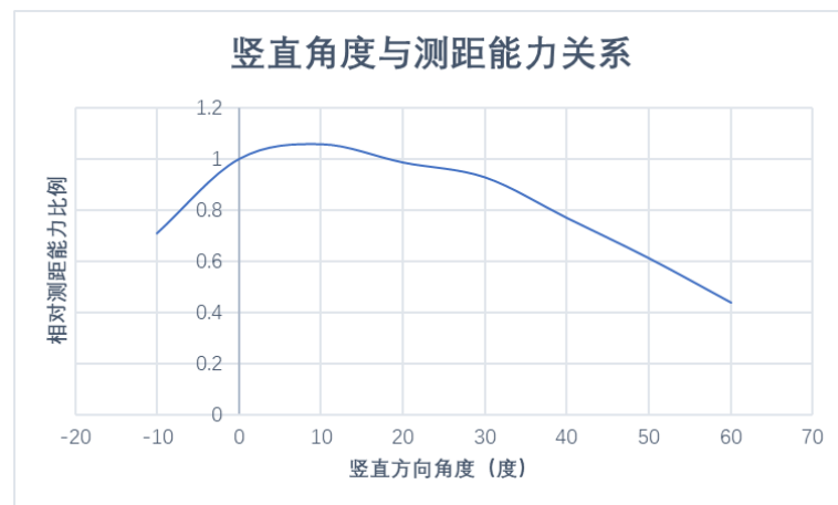
LDS-M300-E-3 不同竖直角测距能力
