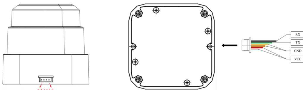
图 5-1 接口定义图
