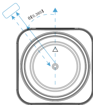
图 5-2 雷达零位及旋转方向示意图
