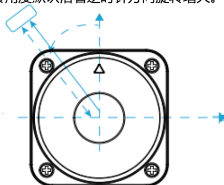
图 5-2 雷达零位及旋转方向示意图
