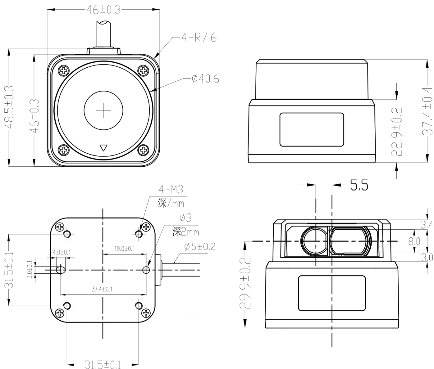
图 4-1 外观及内部结构尺寸示意图
