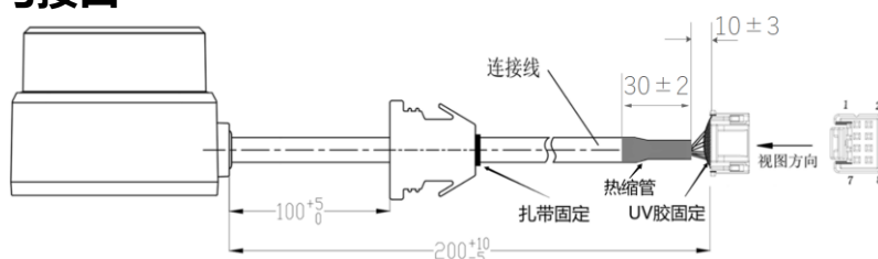
图 5-1 接口定义图
