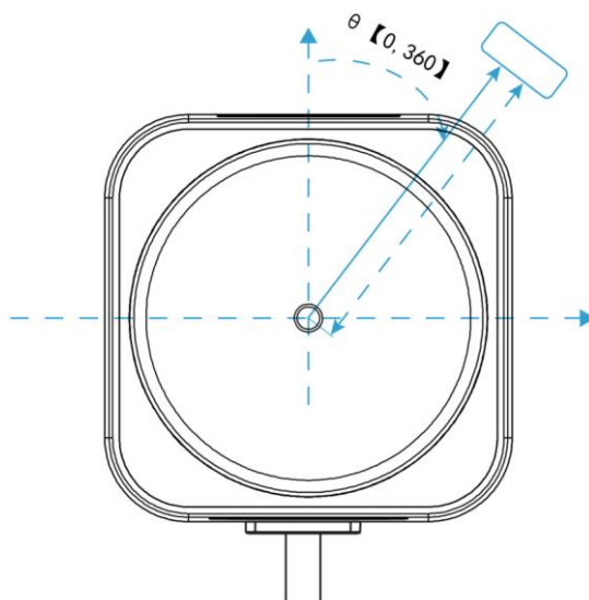
图 5-2 雷达零位及旋转方向示意图
