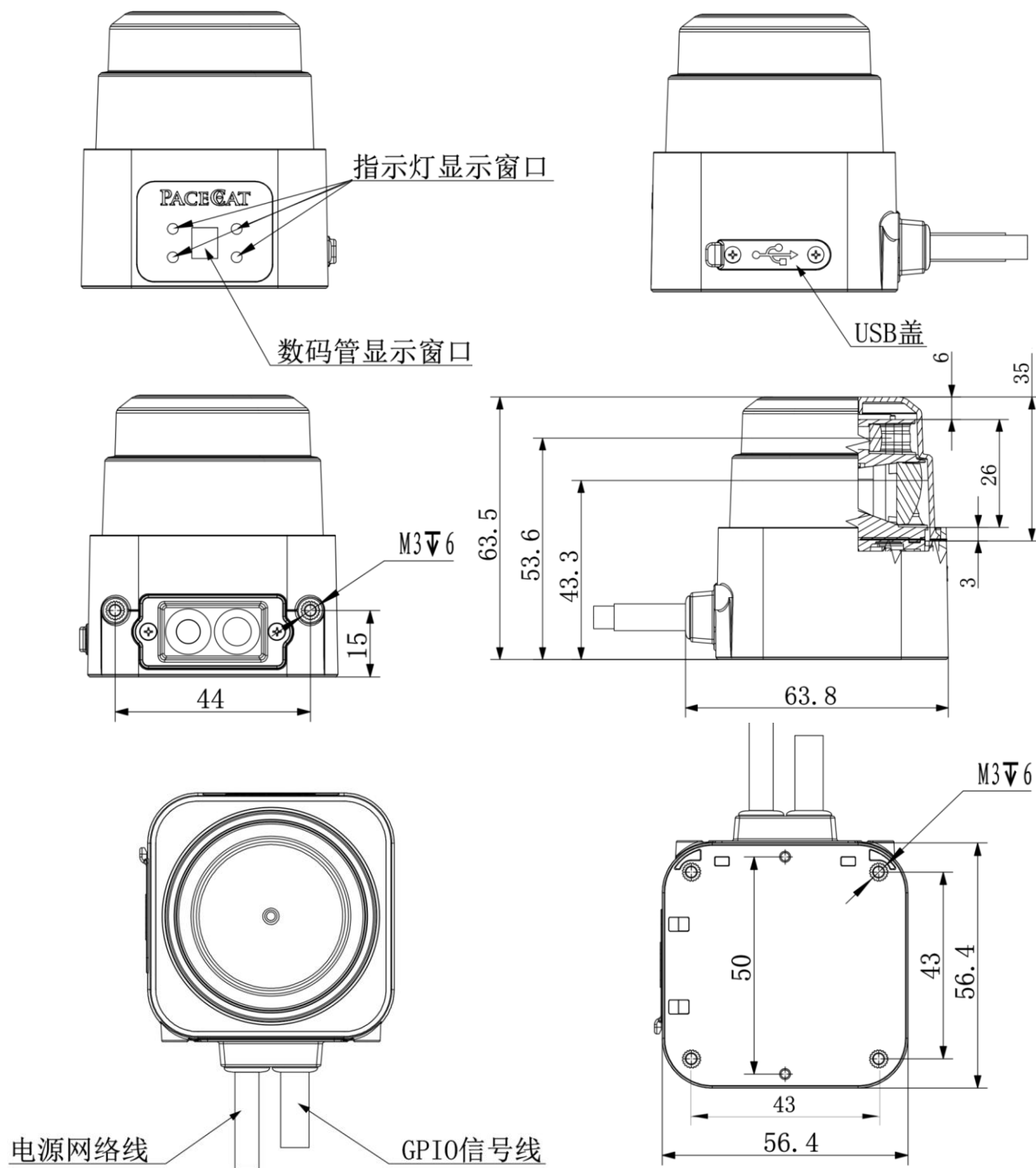
图 4-1 外观及内部结构尺寸示意图
